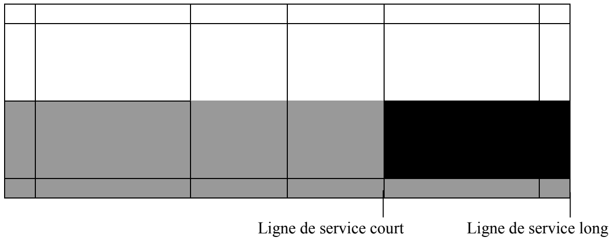
Terrain et zone de service pour le jeu de Simples badminton sous la taille classe 1 & 2
