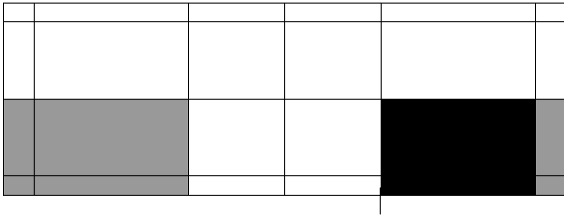
Ligne de service court Ligne de service long Terrain et zone de service pour le jeu de Simples badminton en fauteuil classe 3 – BMW3
