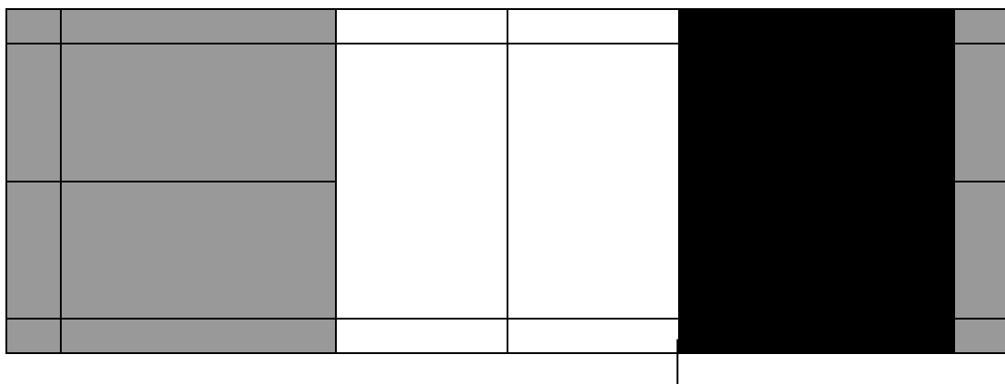
Ligne de service court Ligne de service long Terrain et zone de service pour le jeu de Doubles badminton en fauteuil classe 3– BMW 3
